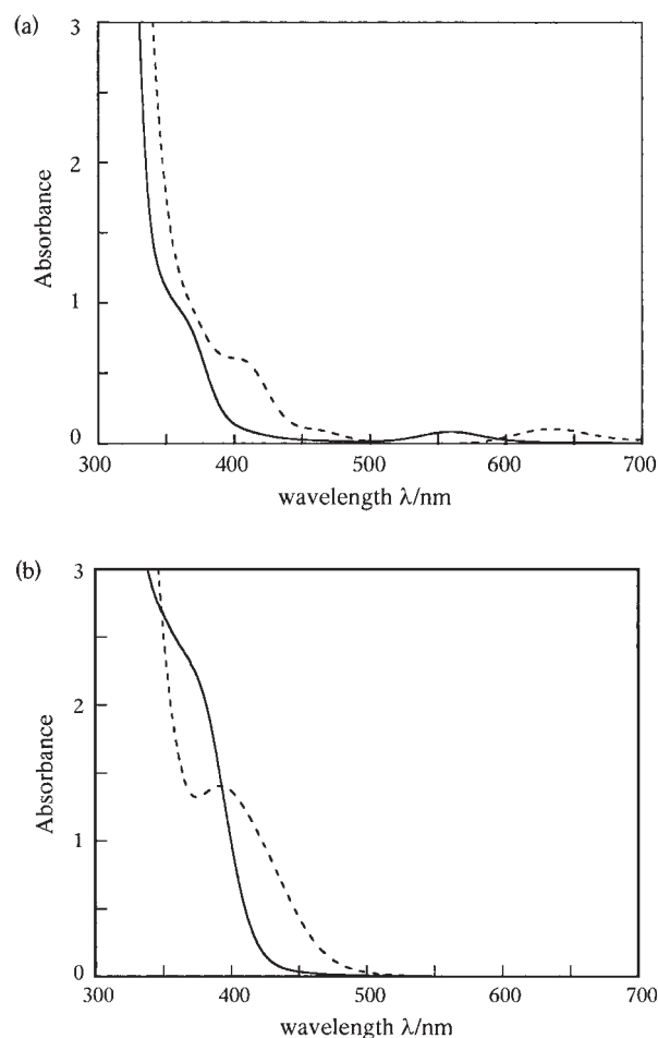
Fig. 4. Electronic spectra in CH 2 Cl 2 solution of (a) 4b (—) and 5b (---), (b) 6 (—) and 7 (---).
